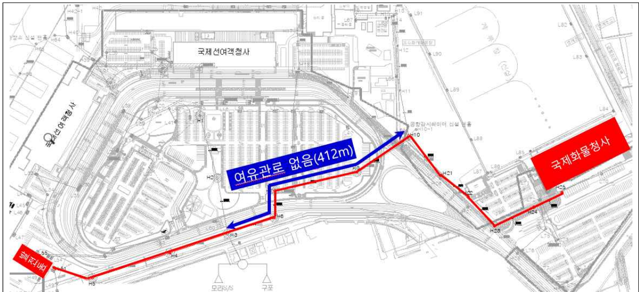
【그림】 김해공항 관로현황(발전동 ~ 국제화물청사)
