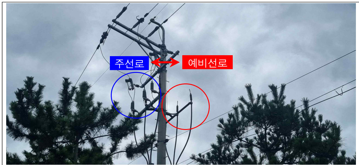
【그림2】 한전인입전주 현황
